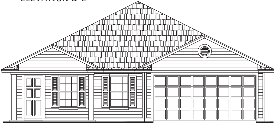
ELEVATION D-3
